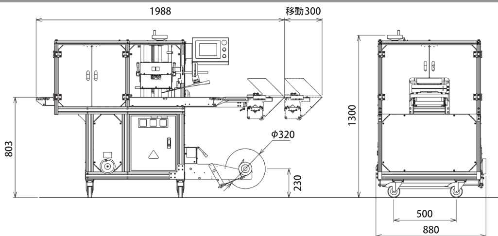
FR-110 製品外寸
